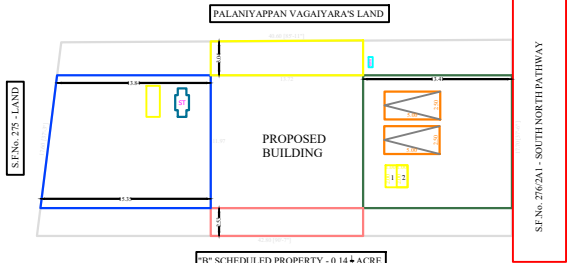
SITE PLAN (SCALE - 1:200)
