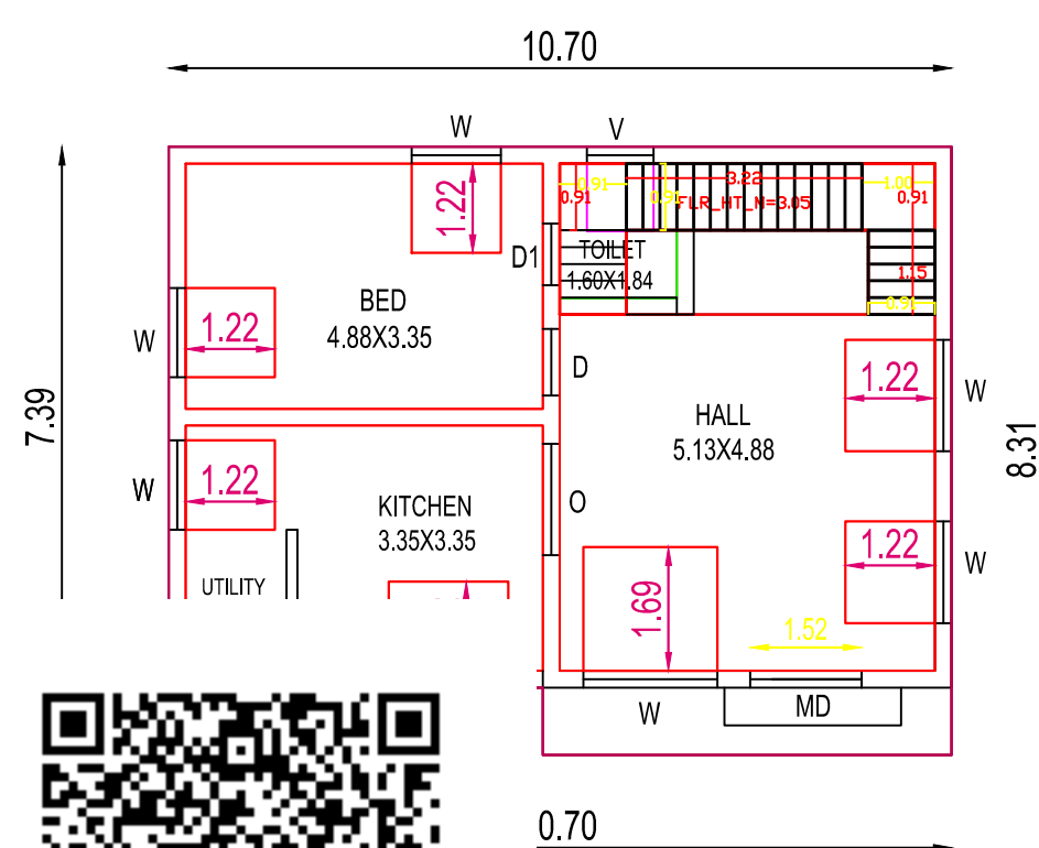
FLOOR PLAN e 1:100)
