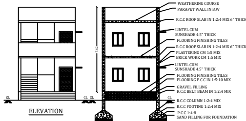
SECTION A-B
