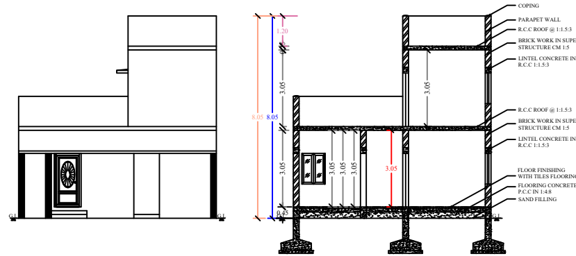
ELEVATION
