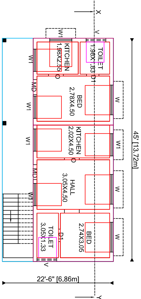
PLAN.
