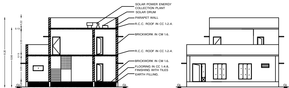
SECTION A-B
