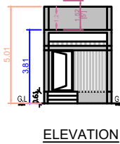
ELEVATION
