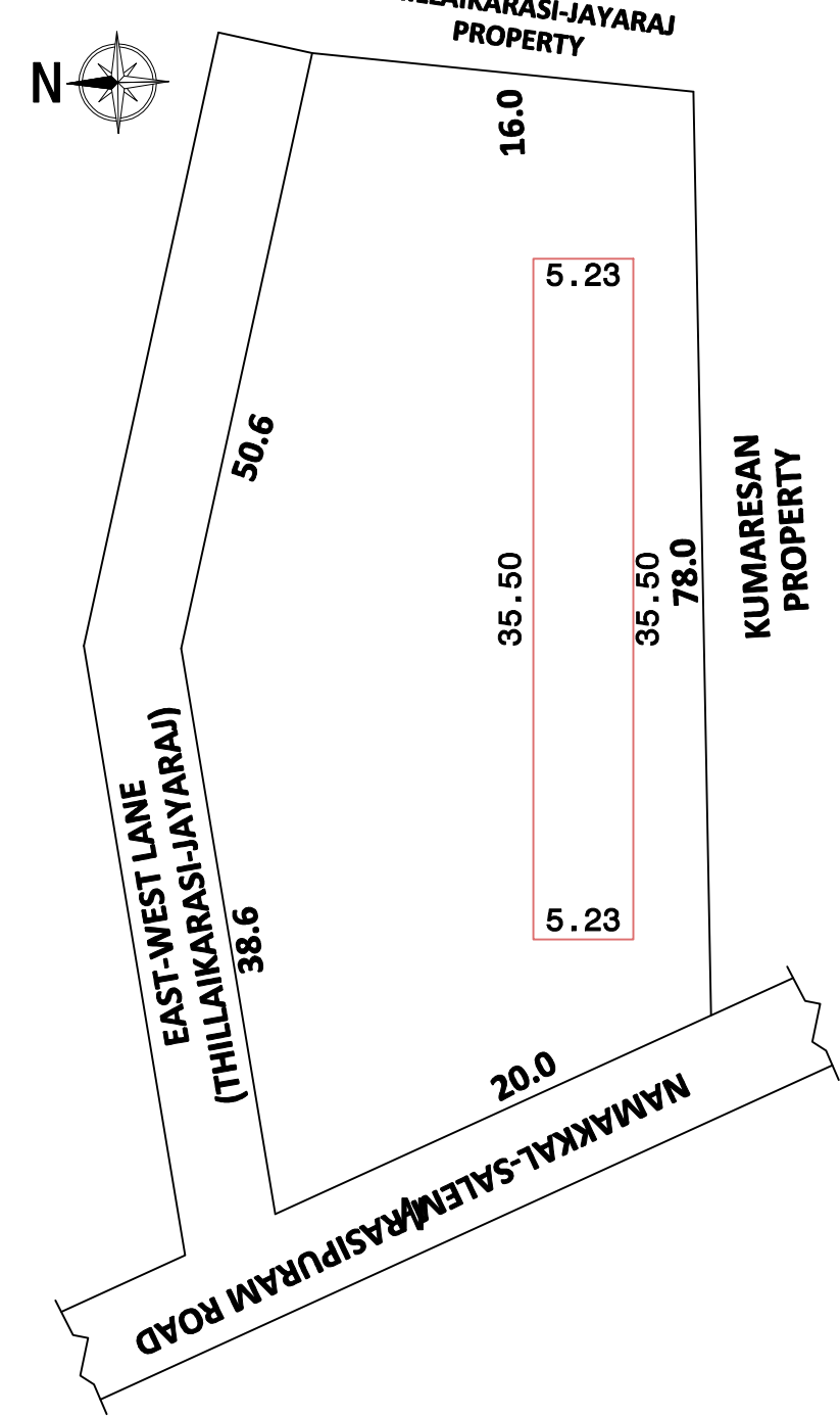
SITE PLAN Scale - 1:600
