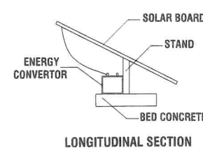
LONGITUDINAL SECTION
