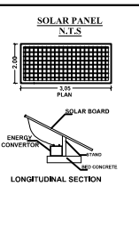
LONGITUDINAL SECTION
