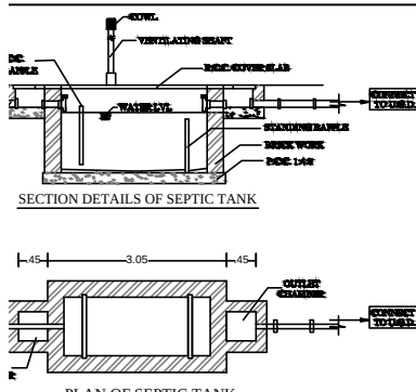
TAILS OF SEPTIC TANK (N.T.S.)
