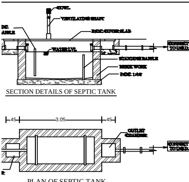
DETAILS OF SEPTIC TANK (N.T.S.)
