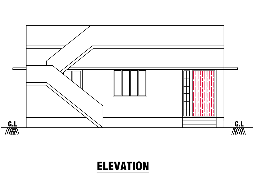
ELEVATION
