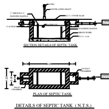
DETAILS OF SEPTIC TANK (N.T.S.)
