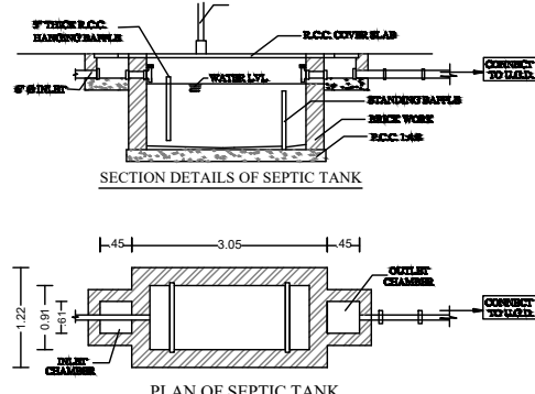
DETAILS OF SEPTIC TANK (N.T.S.)
