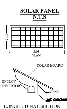
LONGITUDINAL SECTION
