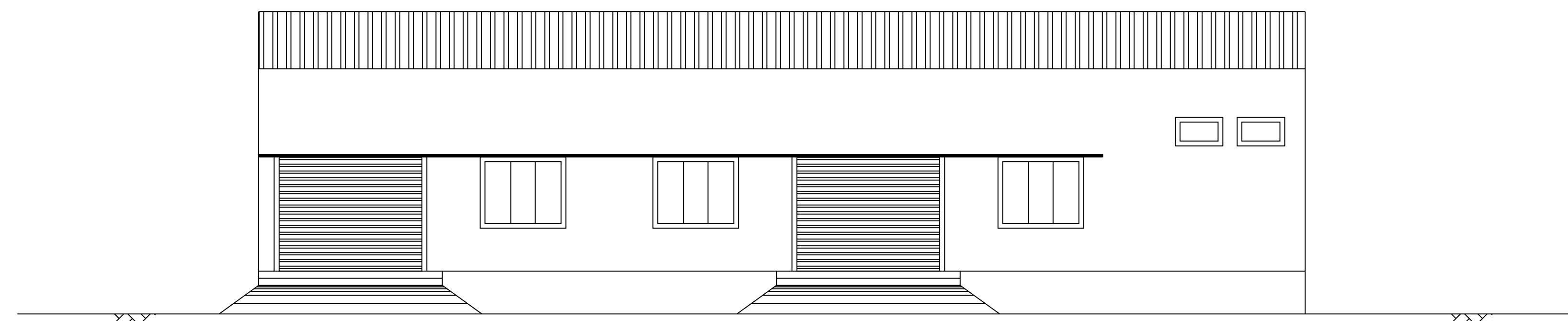
ELEVATION
