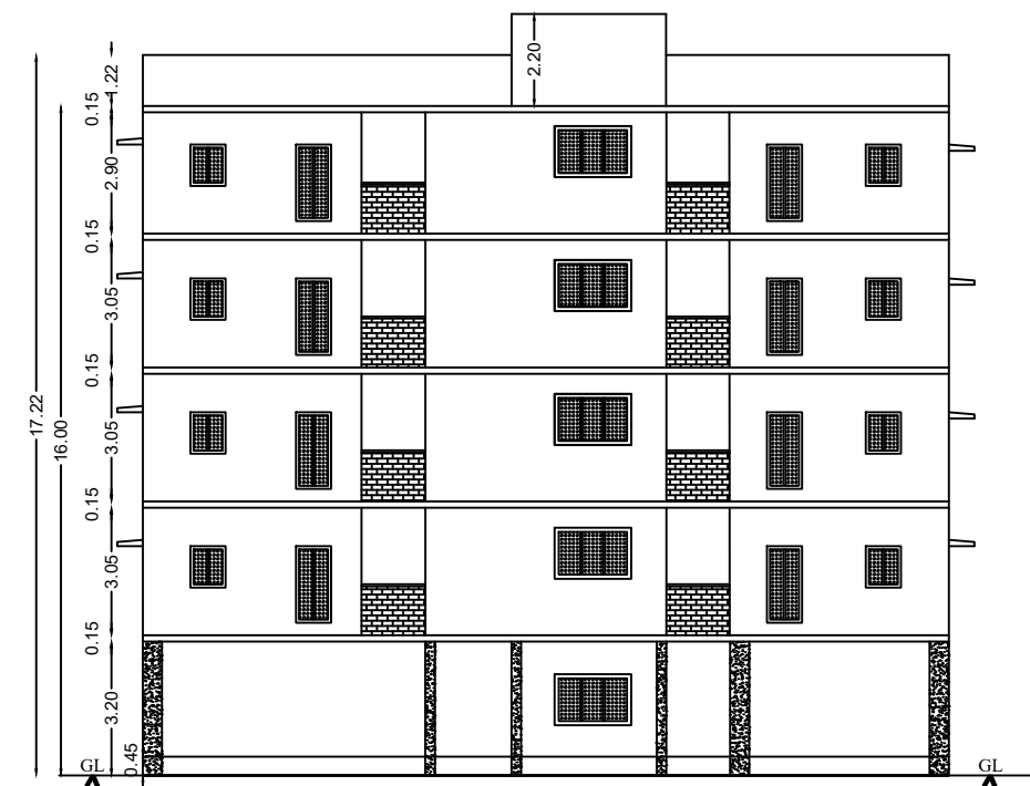
ELEVATION
