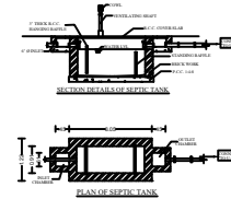
DETAILS OF SEPTIC TANK (N.T.S.)
