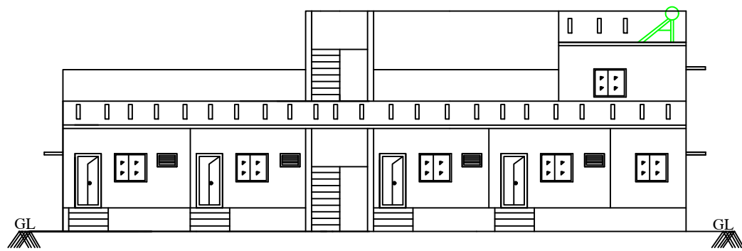
ELEVATION
