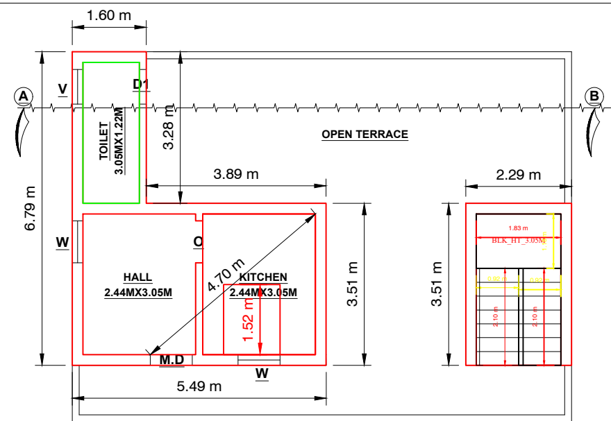
S.F PLAN
