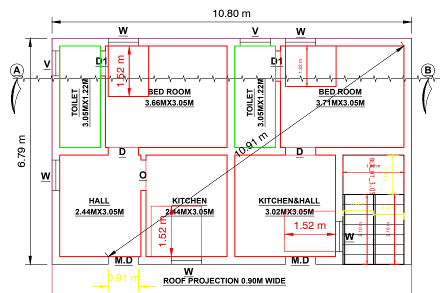
G.F PLAN
