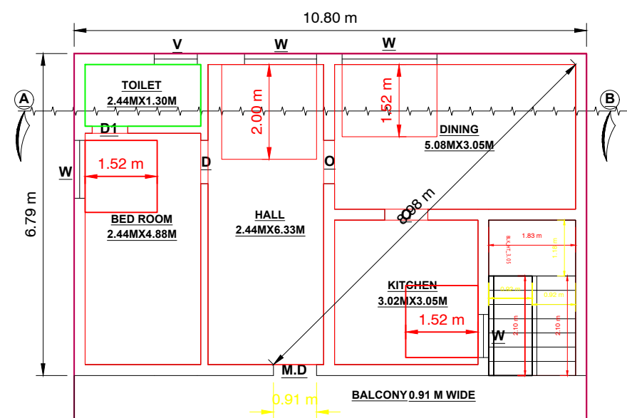
F.F PLAN
