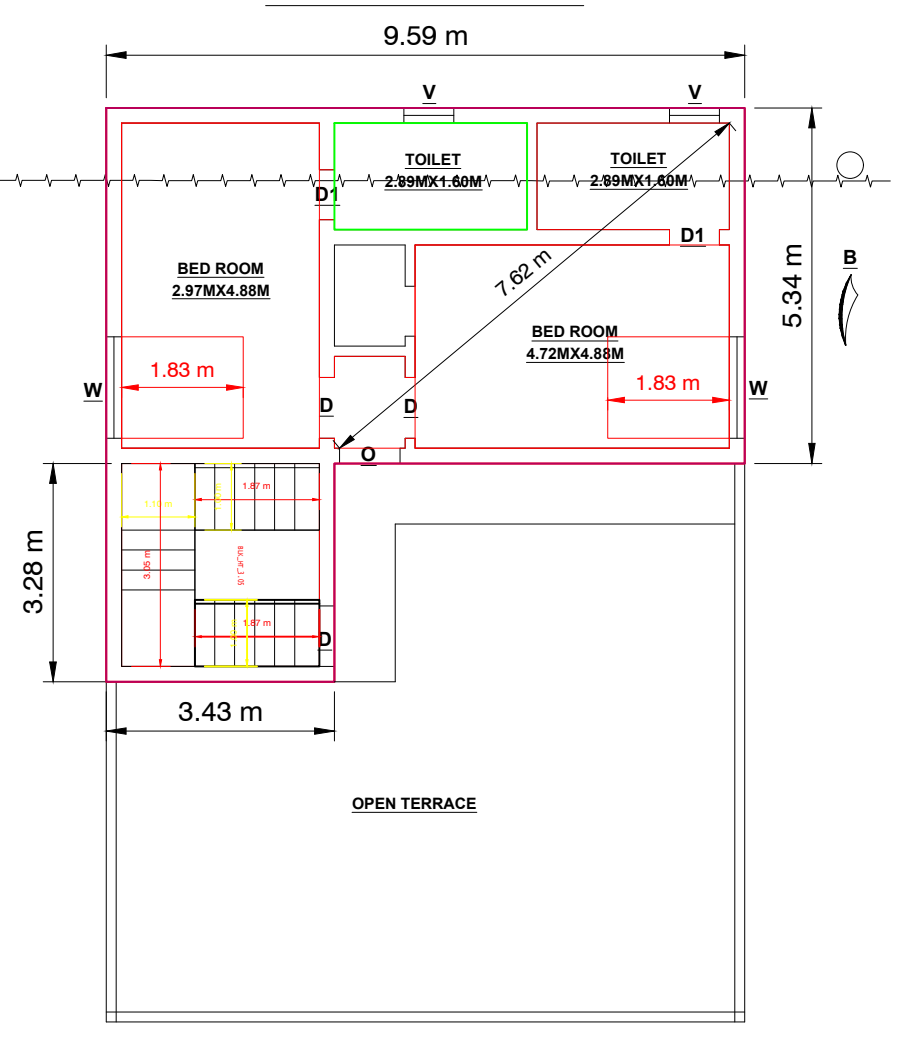
F.F PLAN
