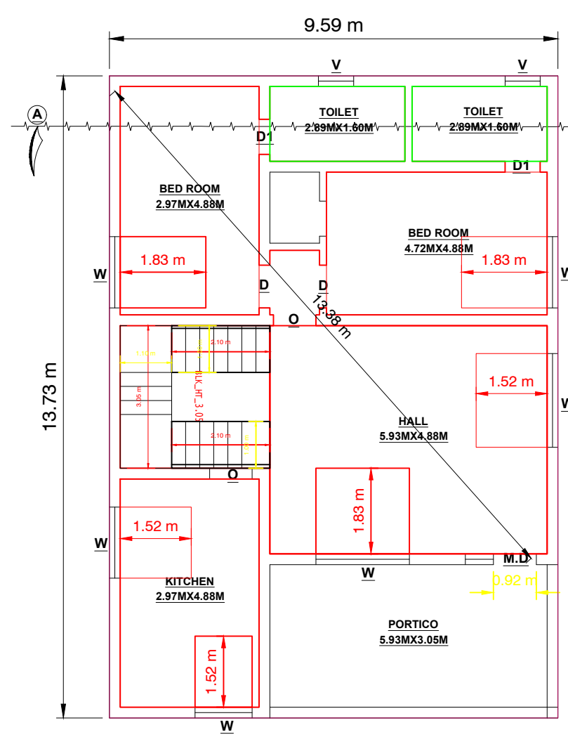
G.F PLAN
