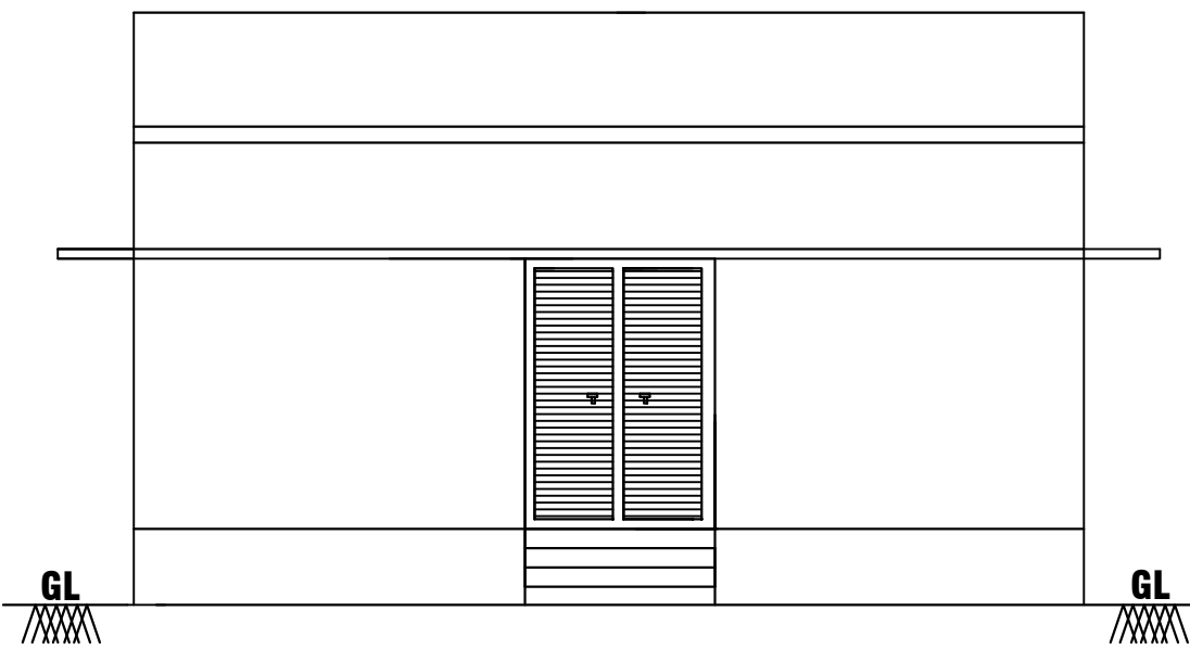
ELEVATION
