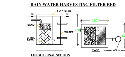
LONGITUDINAL SECTION
