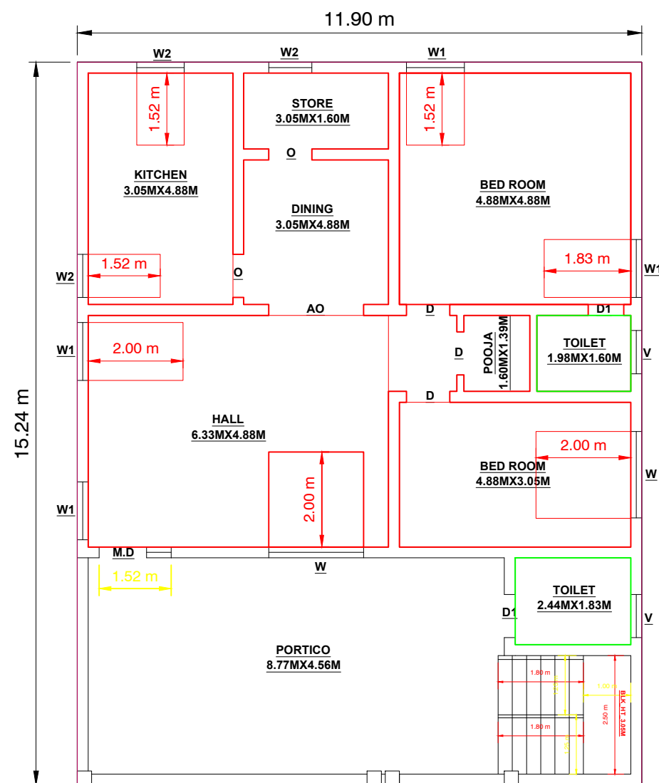
G.F PLAN
