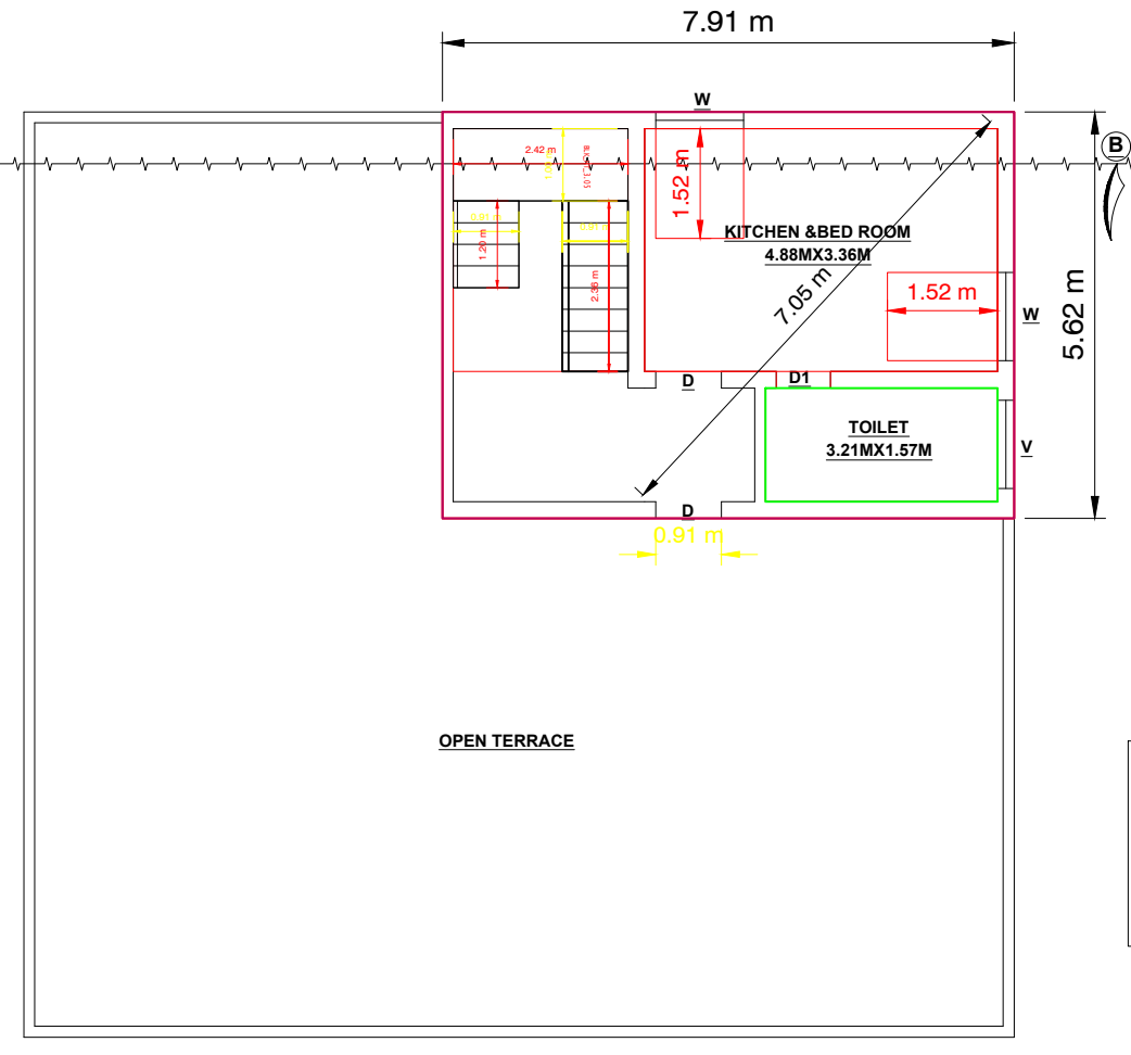
F.F PLAN
