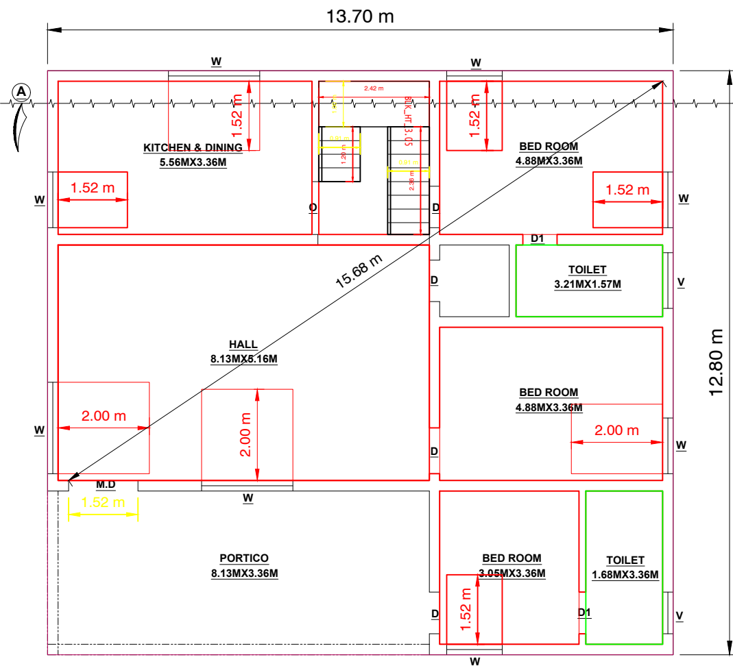
G.F PLAN
