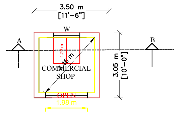
PLAN ( SCALE 1 : 100 )
