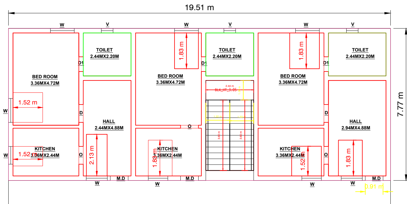
G.F PLAN
