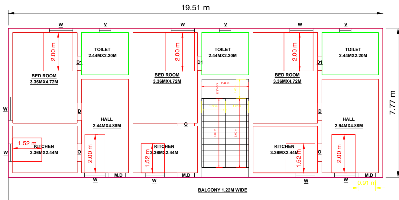
F.F PLAN
