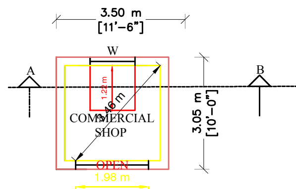
PLAN ( SCALE 1 : 100 )
