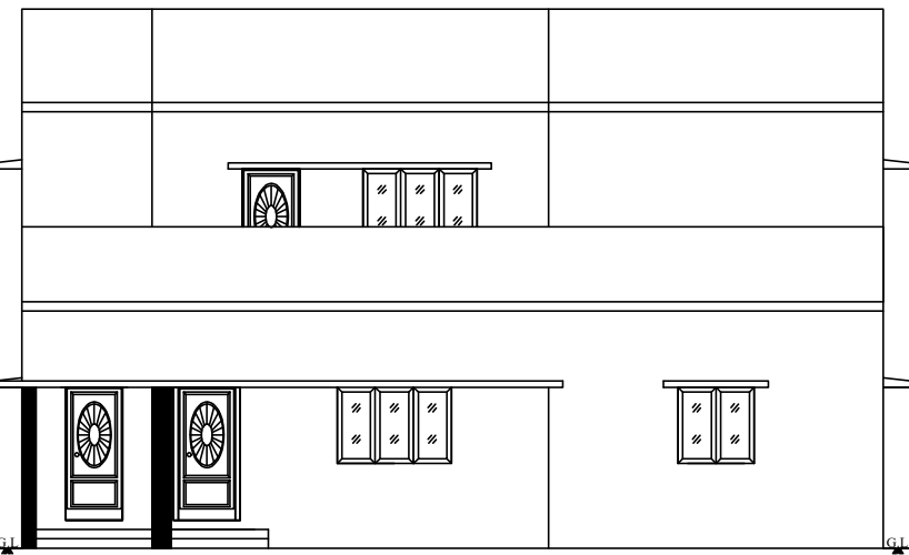
ELEVATION
