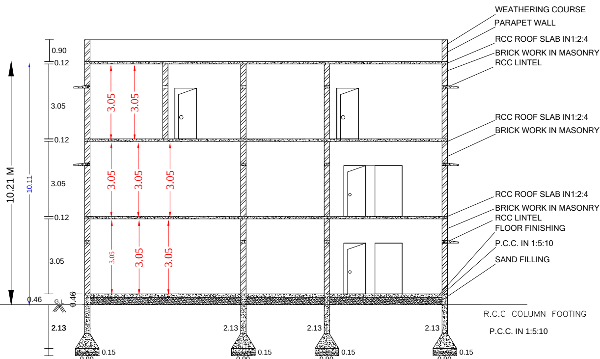
SECTION - AB
