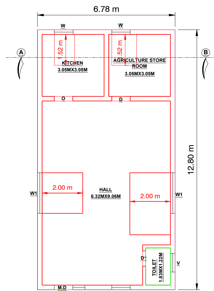
G.F PLAN
