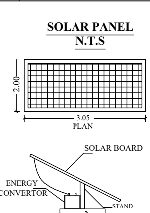
LONGITUDINAL SECTION
