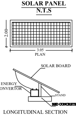
LONGITUDINAL SECTION
