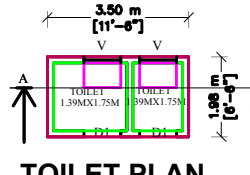
TOILET PLAN
