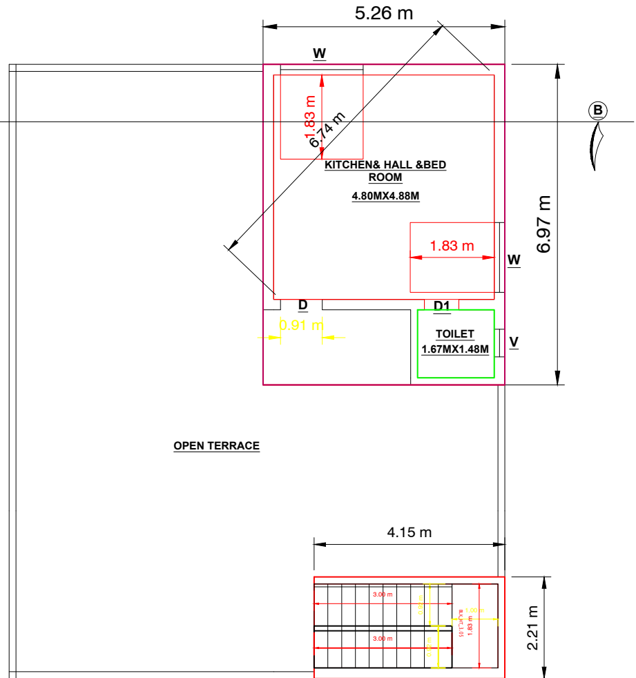
F.F PLAN
