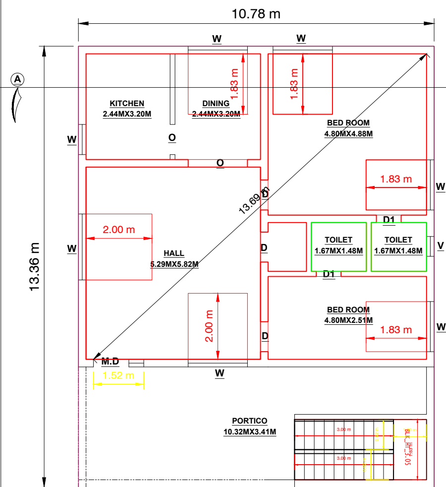
G.F PLAN
