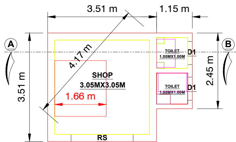
G.F PLAN
