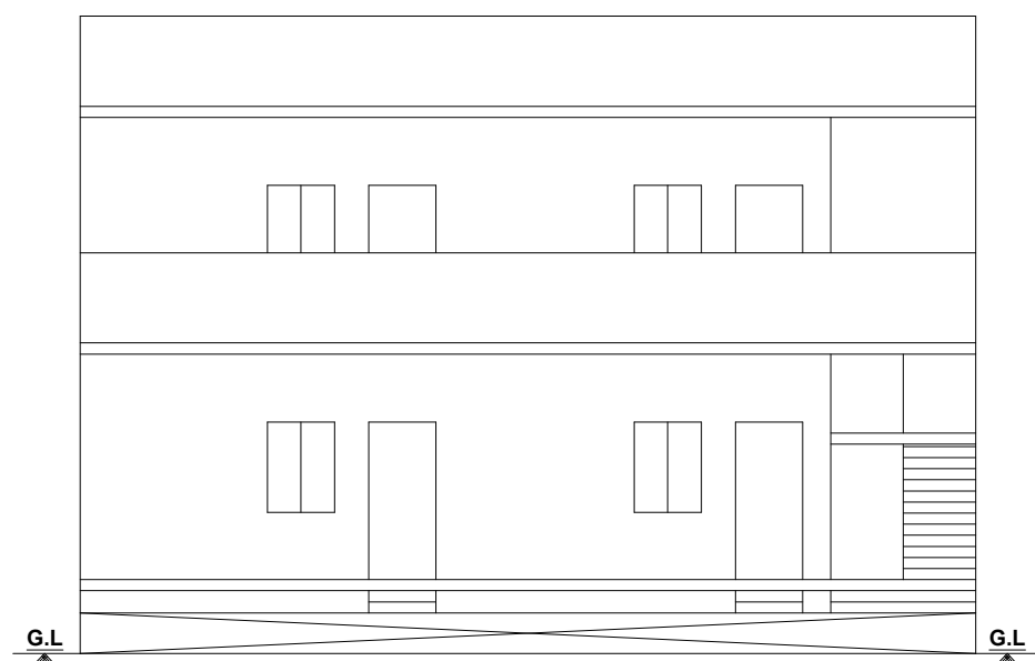
ELEVATION
