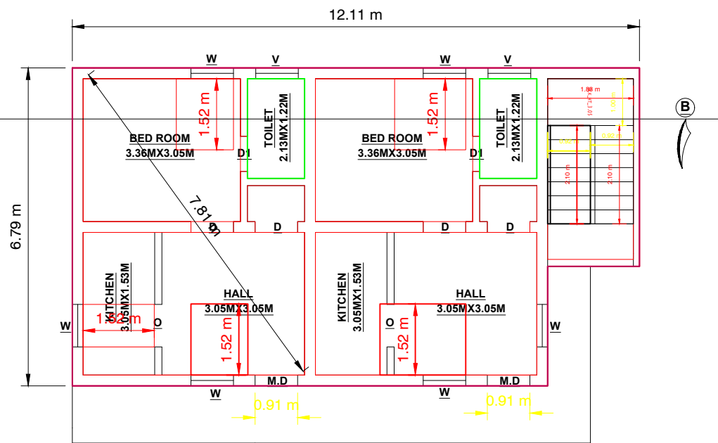
F.F PLAN
