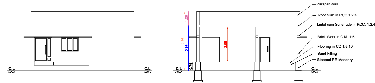
ELEVATION
