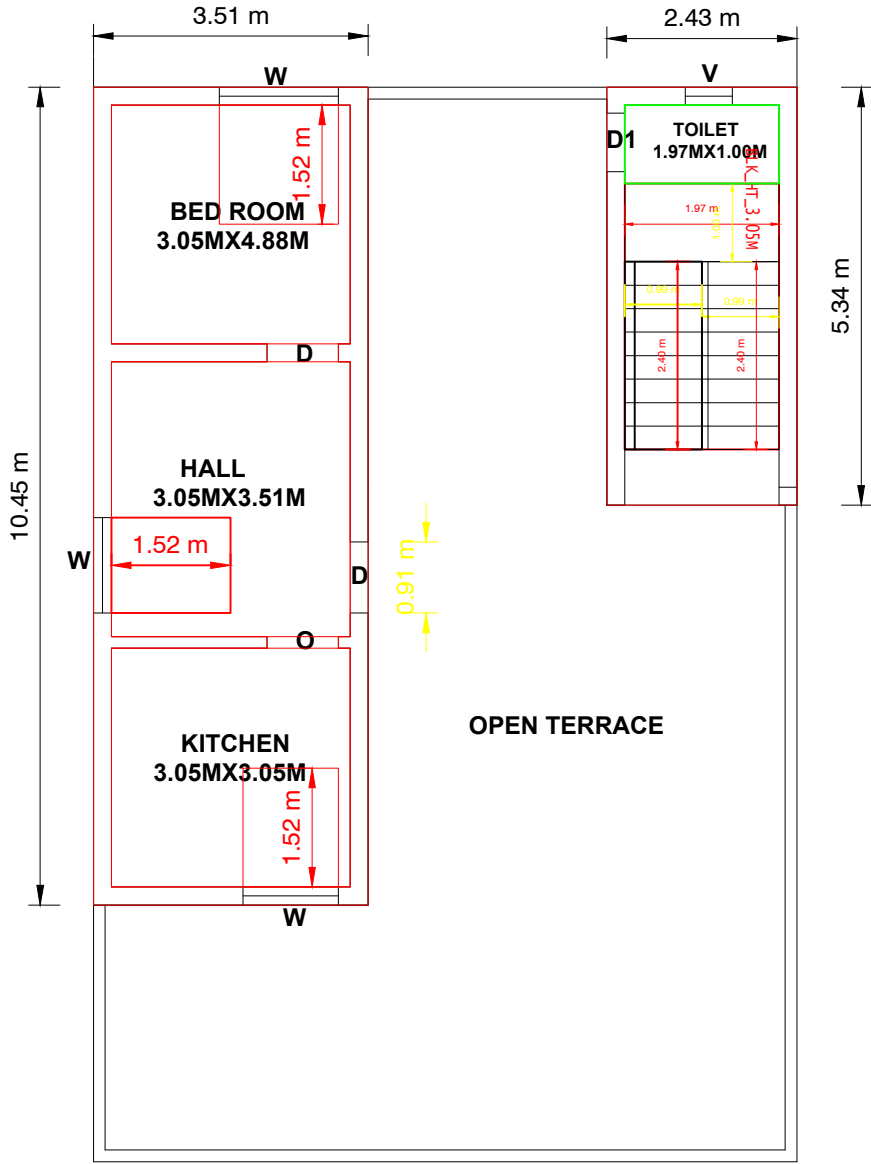
F.F. PLAN
