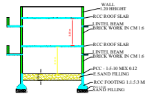
ELEVATION
