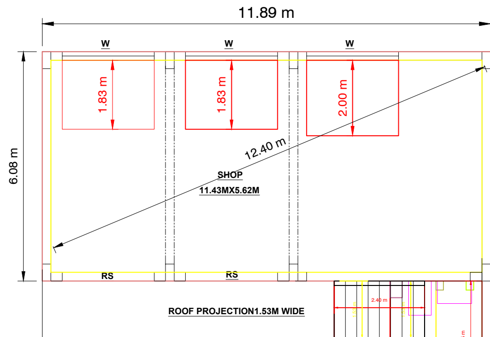
G.F PLAN
