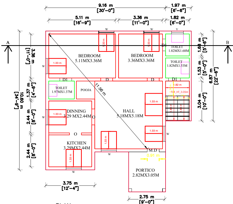
PLAN SCALE ( 1 : 100 )
