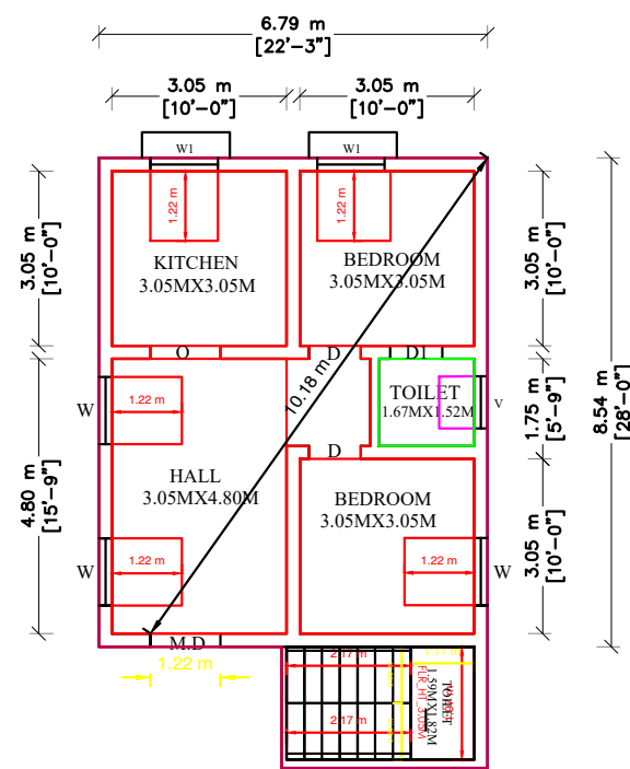
PLAN SCALE ( 1 : 100 )
