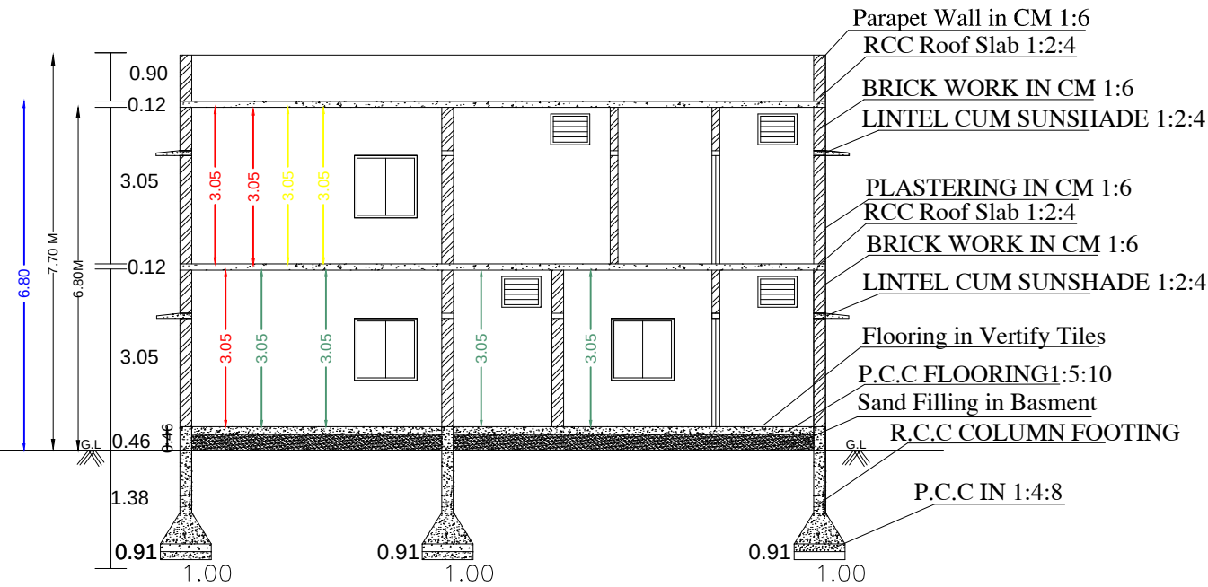
SECTION - AB
