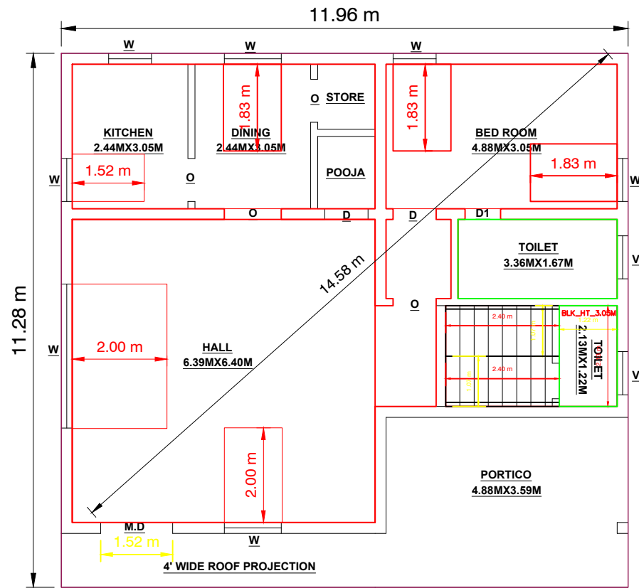
G.F PLAN
