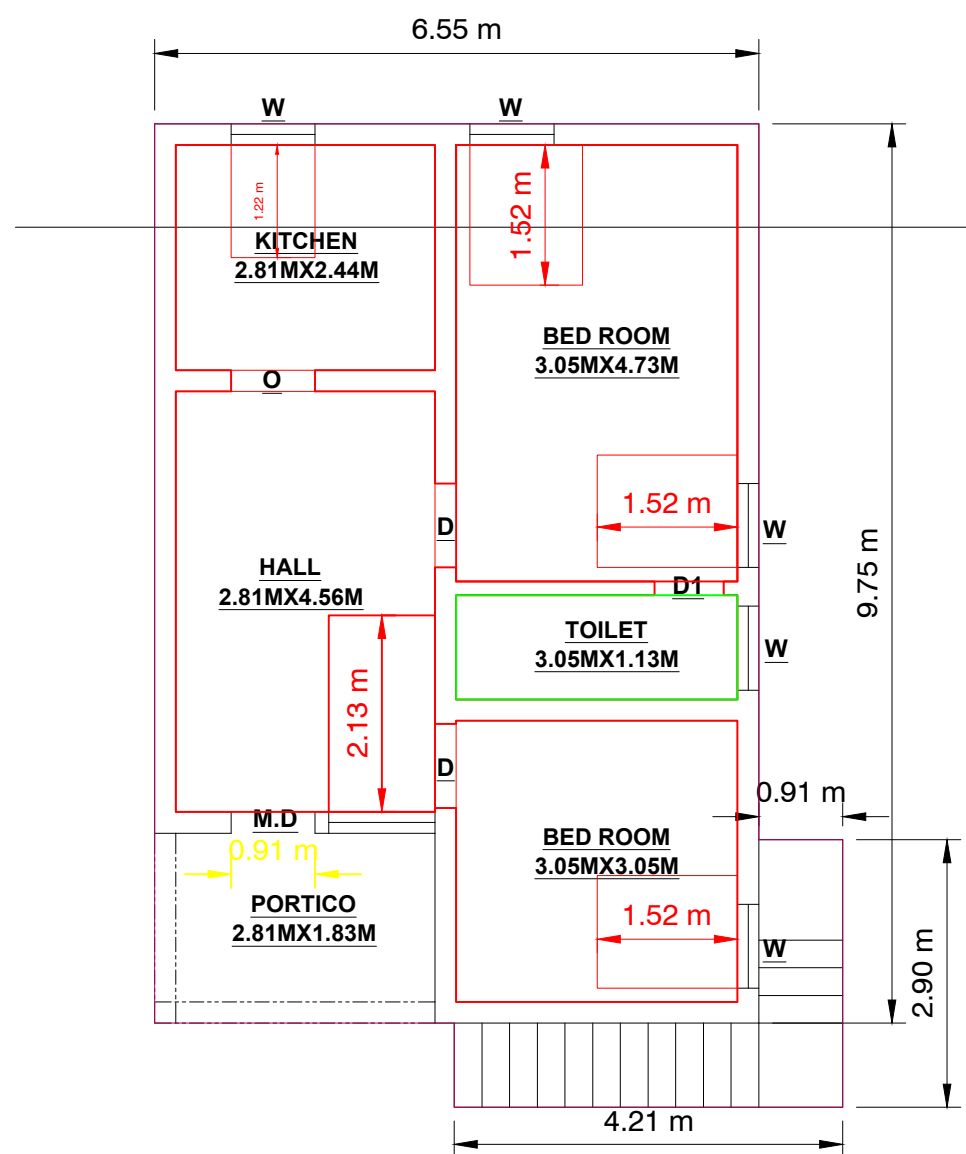
G.F PLAN
