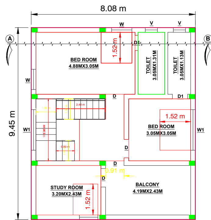
F.F PLAN
