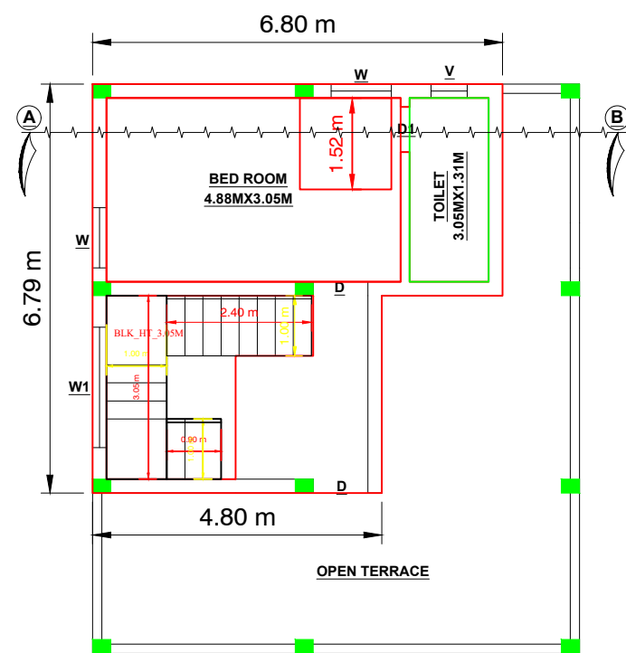
S.F PLAN
