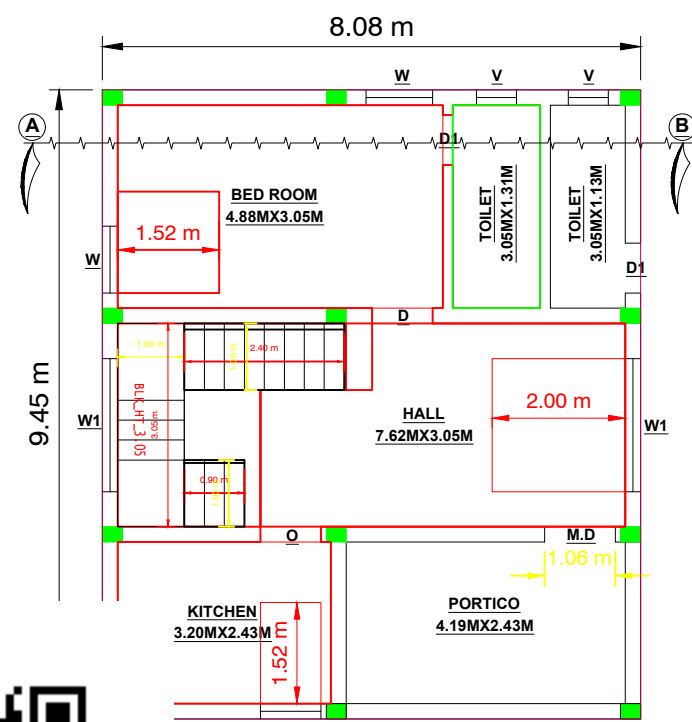
G.F PLAN
