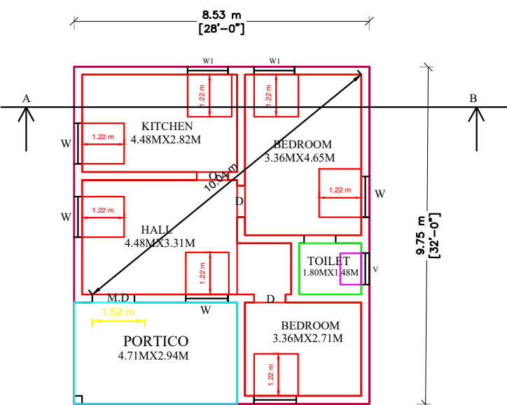
PLAN SCALE ( 1 : 100 )
