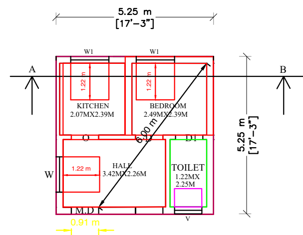
PLAN SCALE ( 1 : 100 )
